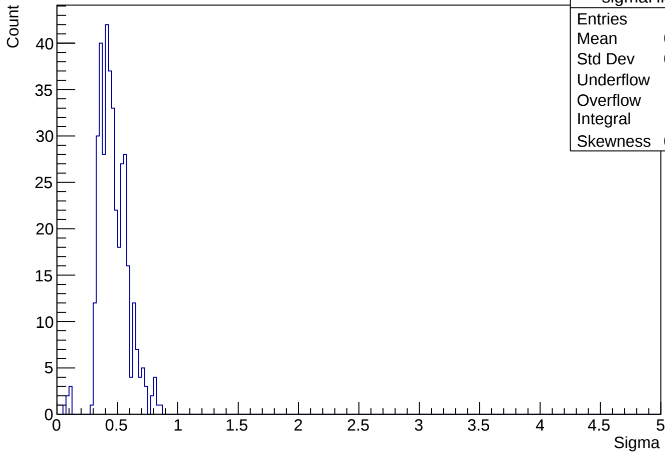
sigmaHisto
