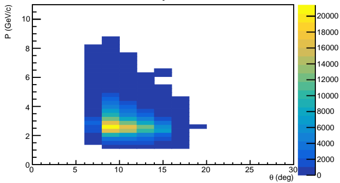
\pi^- layer2
