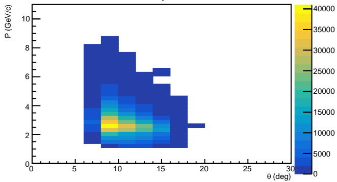
\pi^- layer1
