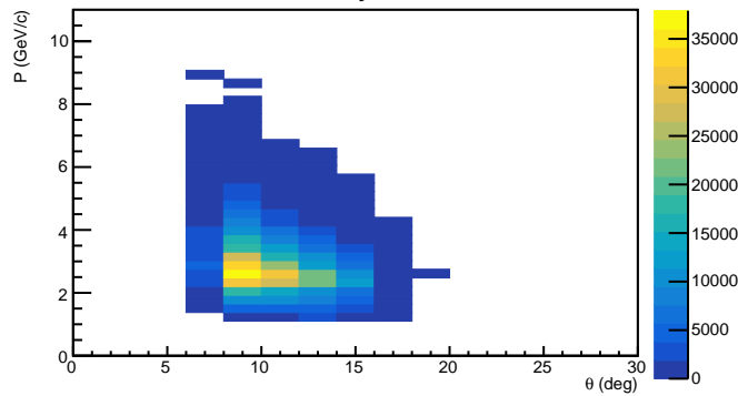
\pi^+ layer1
