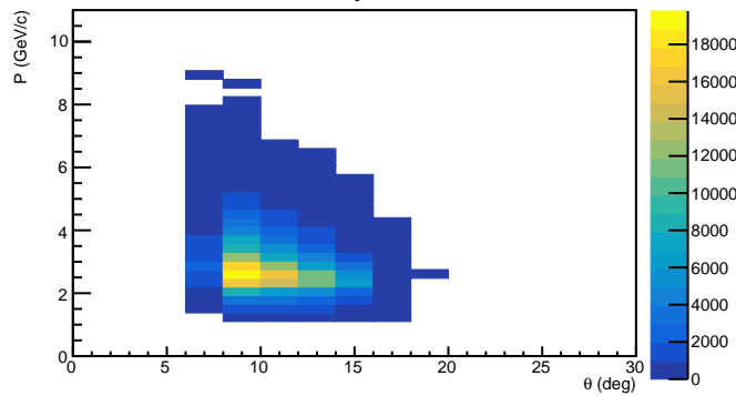
\pi^+ layer2
